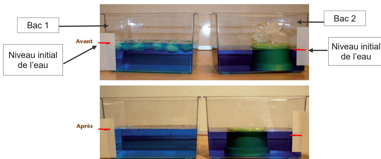
Document 14 - Photographies de l'expérience avant et après la fonte des glaçons (Source : https://fondation-lamap.org/sites/default/files/sequence_pdf/ocean-et-climat-l-augmentation-du-niveau-des-mers.pdf )
