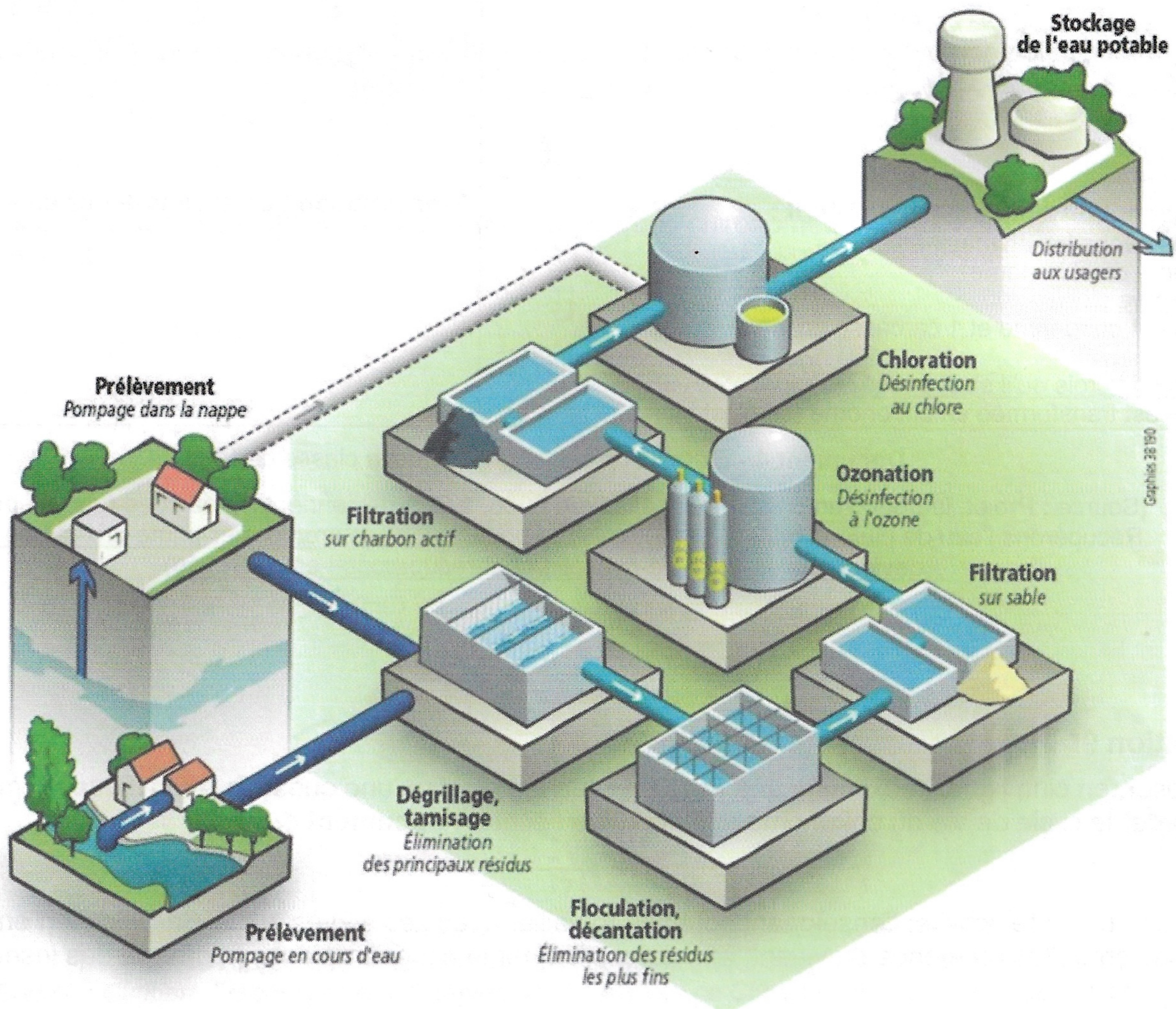
Document 5 - Usine de potabilisation de l'eau
